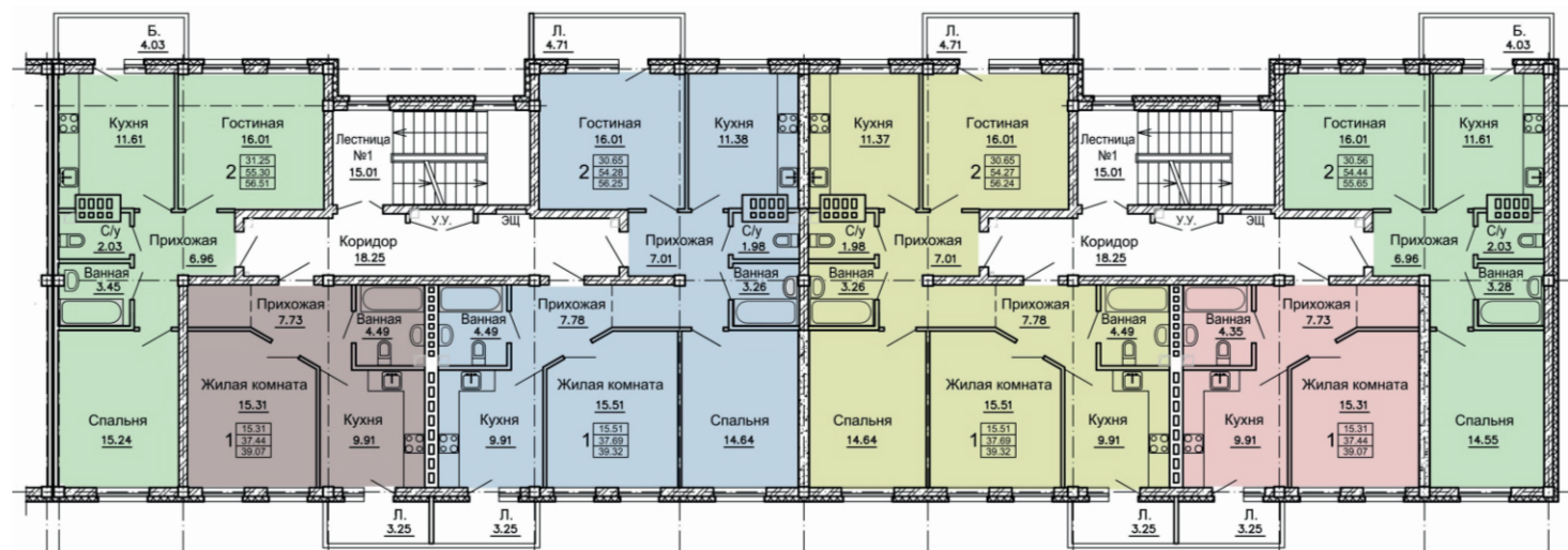
План типовой секции
